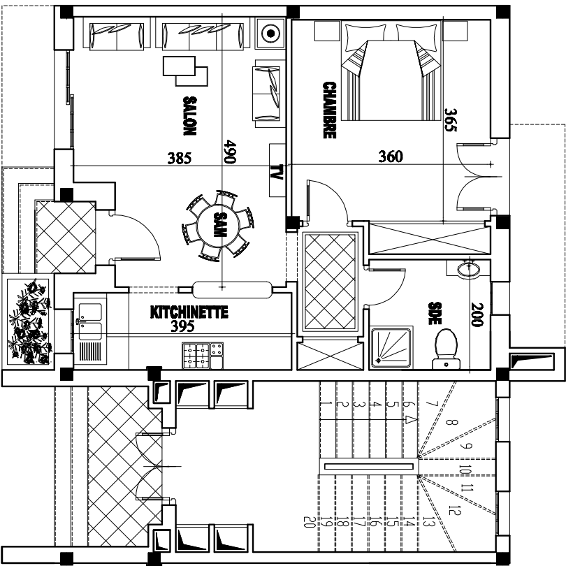
G-2 PLAN RDC
