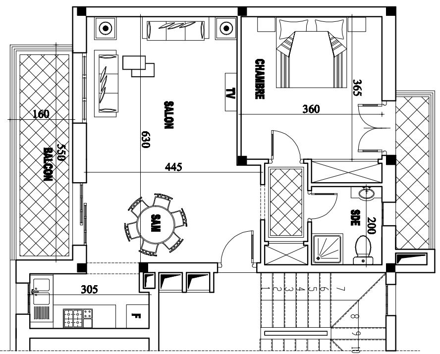
G-2 PLAN RDC
